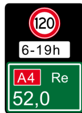
BB07R-A16-52,8 + A1-120-S tussen 6 en 19 h Hectometerbord links met maximale snelheid 120 km/h tussen 9 en 19 h
