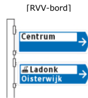
K06 Beslissingswegwijzer langs niet-autosnelweg met interlokale doelen en routenummer niet-autosnelweg
